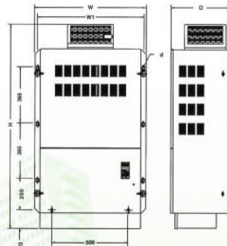
(盘外壁挂型—NEMA1)
