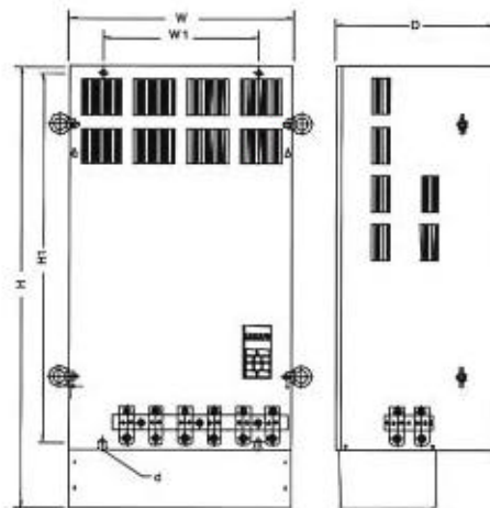
(盘外壁挂型—NEMA1)
