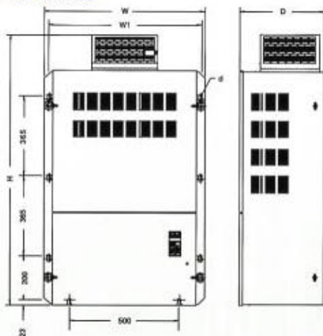
(盘内安装型—IP00)
